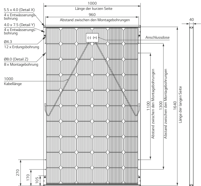
Der Abstand gilt zwischen den Mittelpunkten der Montage- und Erdungsbohrungen.
