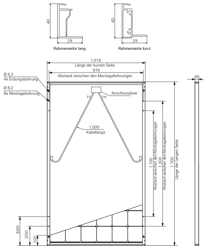
Der Abstand gilt zwischen den Mittelpunkten der Montage- und Erdungsbohrungen.
