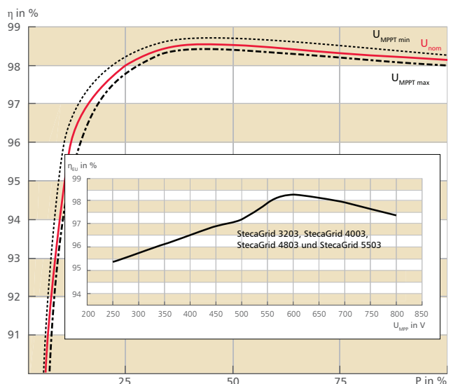
Wirkungsgradverlauf beim StecaGrid 4803 und Vergleich der MPPT-Spannung bei allen Typen
